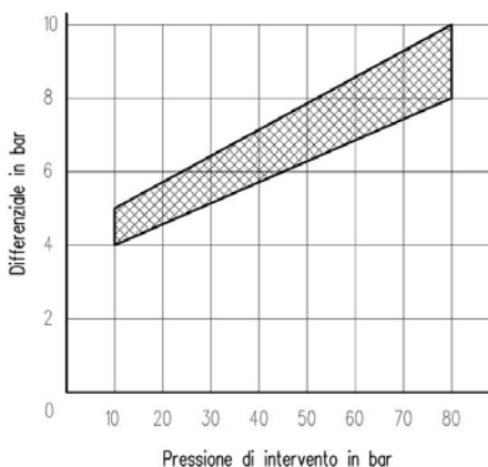
PRESSIONE DIFFERENZIALE DEL PRESSOSTATO IPNB-250
