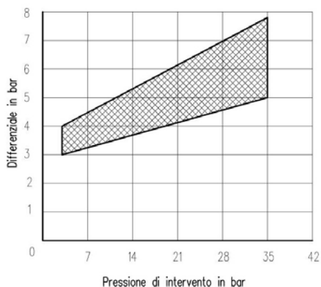
PRESSIONE DIFFERENZIALE DEL PRESSOSTATO IPNB-160
