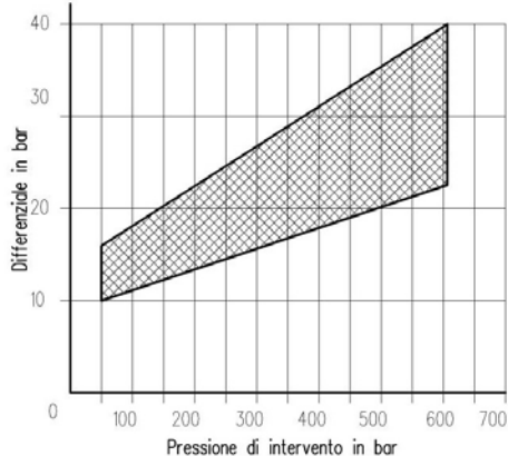
PRESSIONE DIFFERENZIALE DEL PRESSOSTATO IPNB-630
