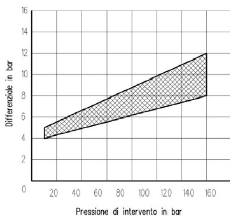
PRESSIONE DIFFERENZIALE DEL PRESSOSTATO IPNB-350
